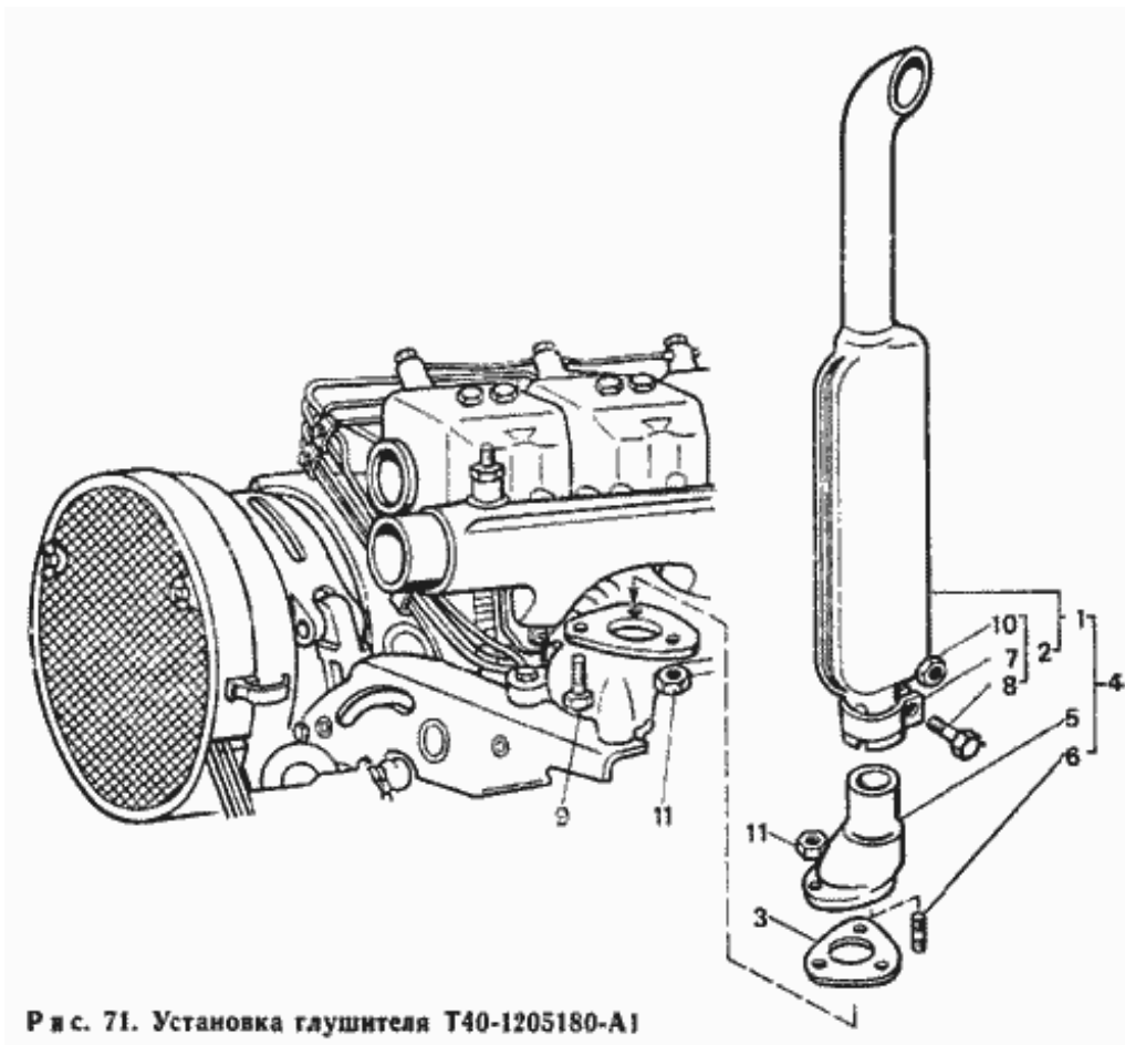
Рис. 071. Установка глушителя Т40-1205180-А1.
